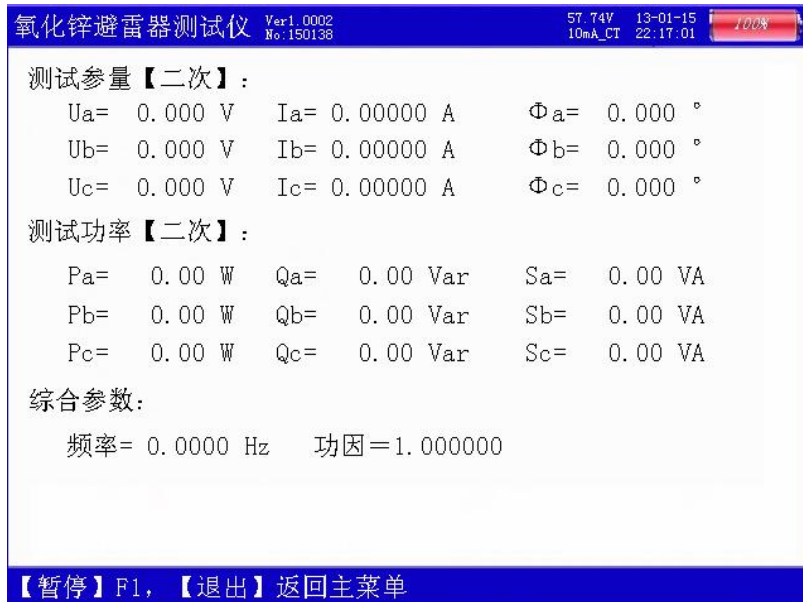
图五、电气测试界面
