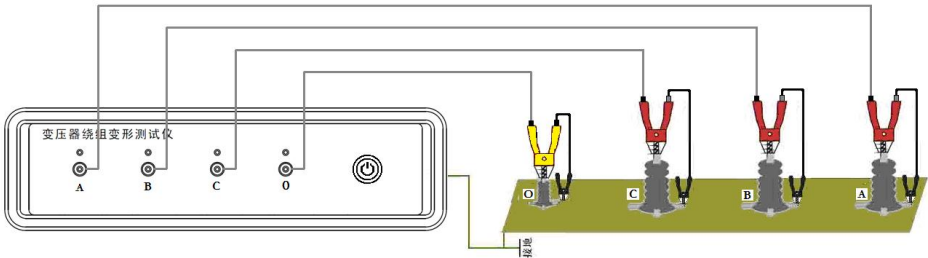
图 2 绕组接线图
