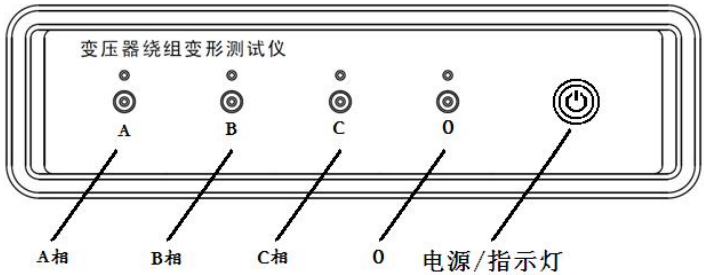
图 1a 变压器绕组变形测试仪面板图(前面板)
